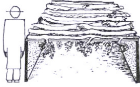
38. היתה גבוהה י' טפחים והוצין יורדין לתוך י'.
